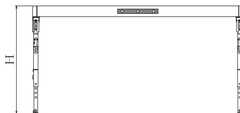
■ 側面図
